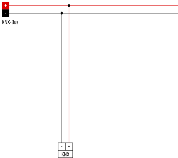
Wiring diagrams
